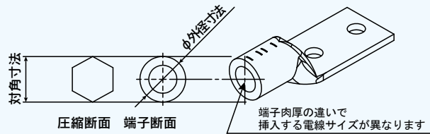
圧縮断面 端子断面
